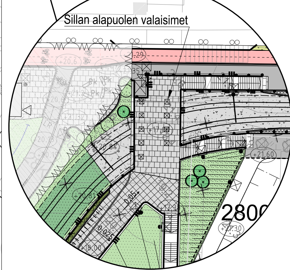
Detalji 1: RAITIOTIESILLAN ALAPUOLI JA YMPÄRISTÖ 1:500
