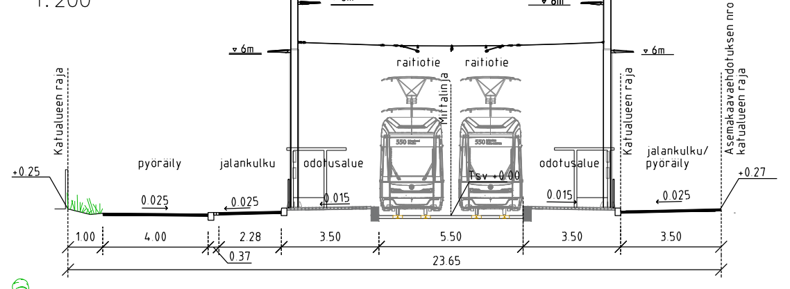
MAAHERRANTIE POIKKILEIKKAUS B - B 1:200
