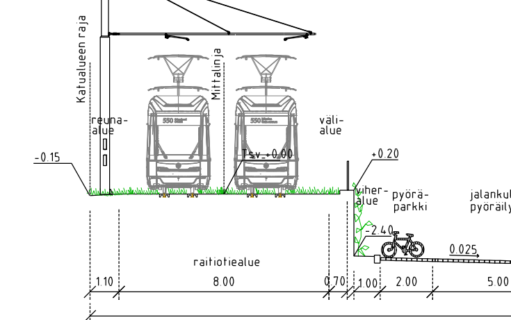
MAAHERRANTIE POIKKILEIKKAUS A - A 1:200
