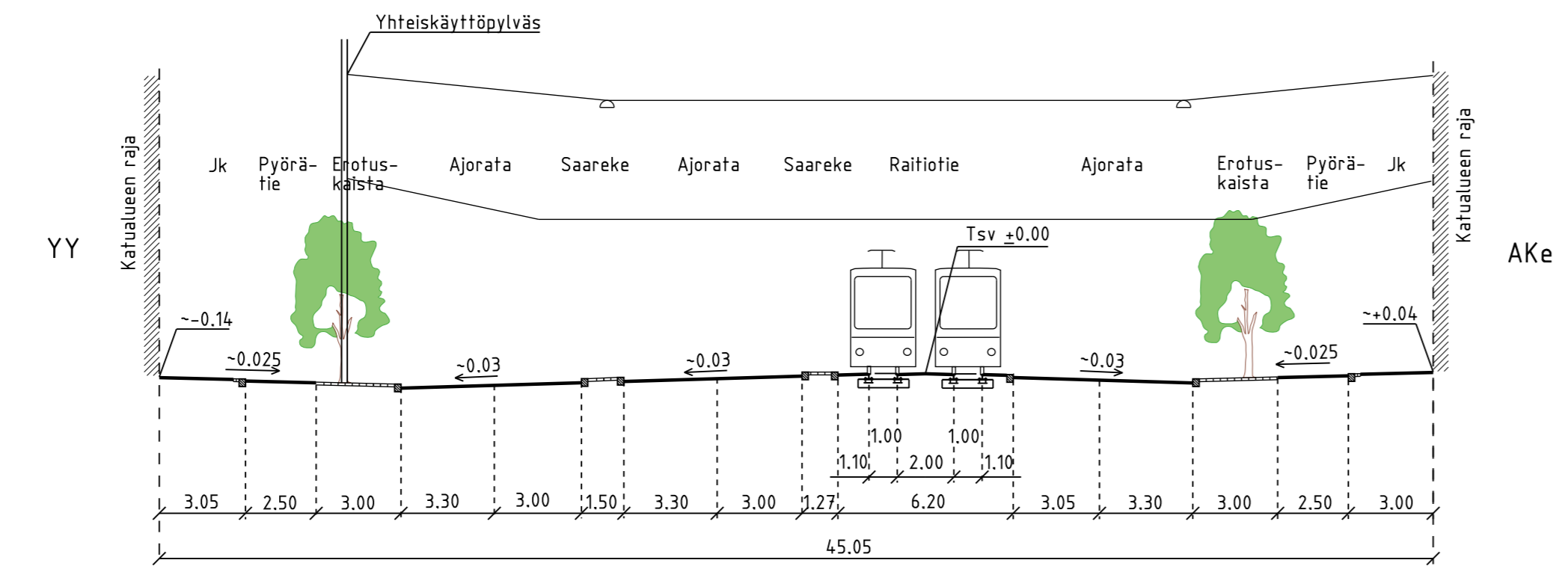
POIKKILEIKKAUS A-A 1:200
