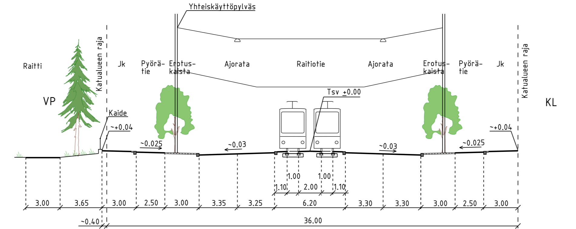
POIKKILEIKKAUS B-B 1:200
