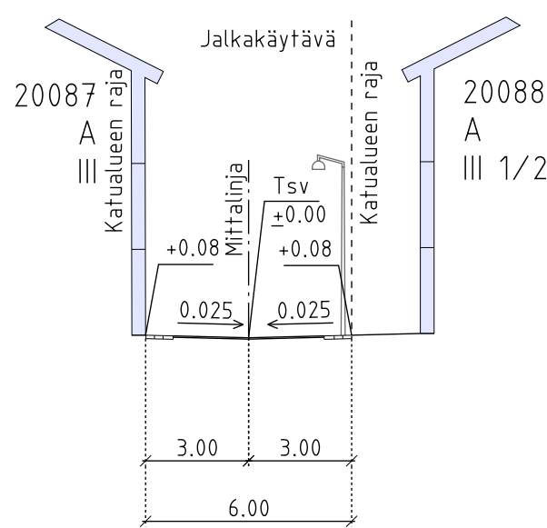
TONGANKUJA LEIKKAUS A-A 1:200
