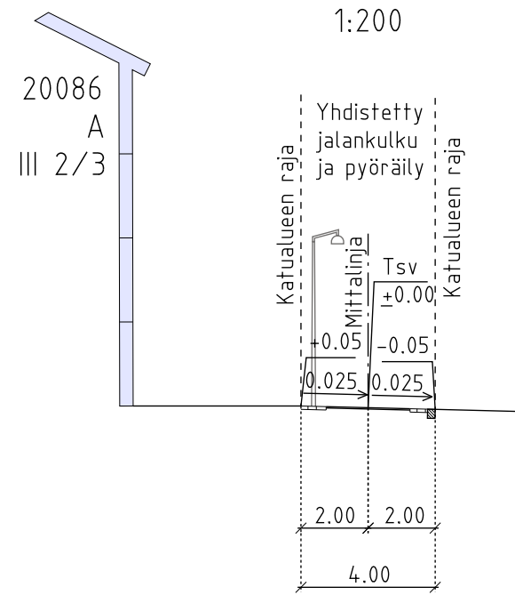
NEPTUNUKSENKUJA LEIKKAUS A-A 1:200
