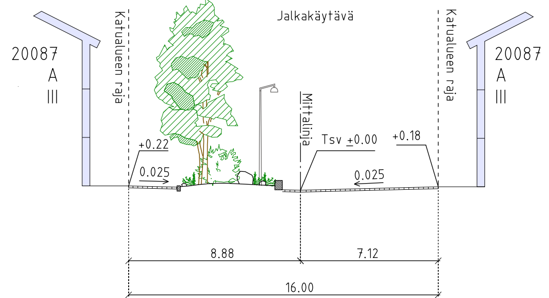
TONGANKUJA LEIKKAUS B-B 1:200
