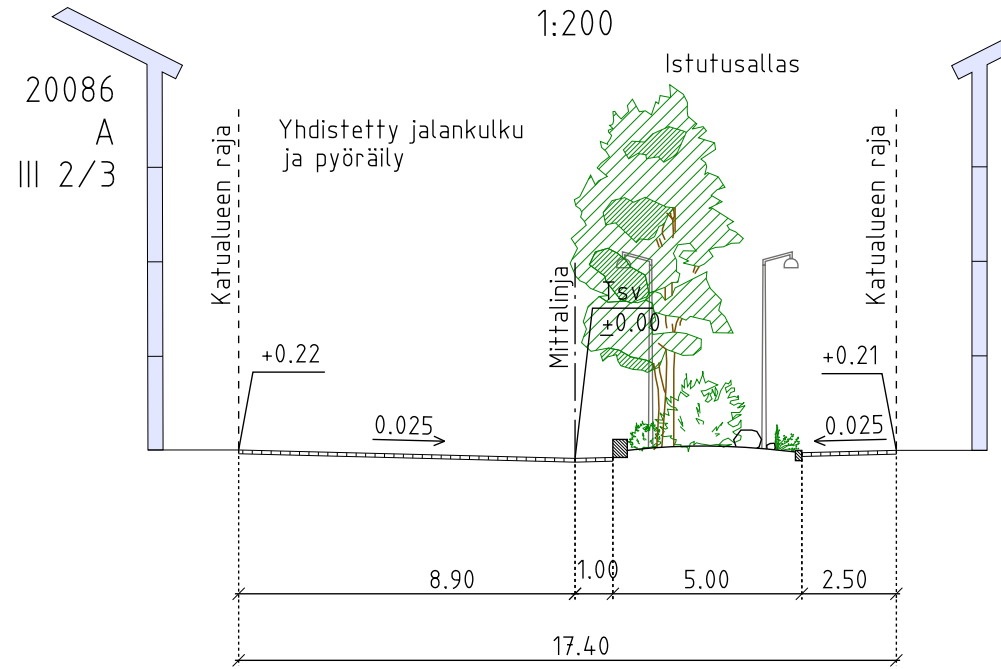
SAMOANKUJA LEIKKAUS A-A 1:200
