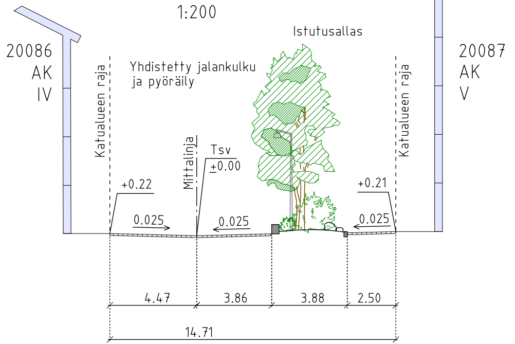
SAMOANKUJA LEIKKAUS B-B 1:200
