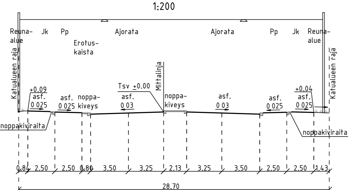
POIKKILEIKKAUS B-B Sturenkatu 1:200
