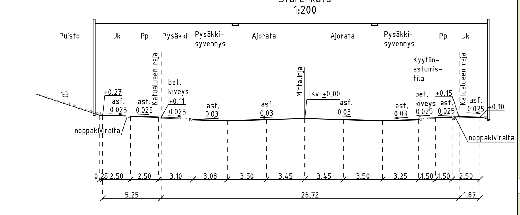
POIKKILEIKKAUS A-A Sturenkatu 1:200
