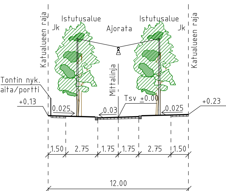
POIKKILEIKKAUS B-B 1:200
