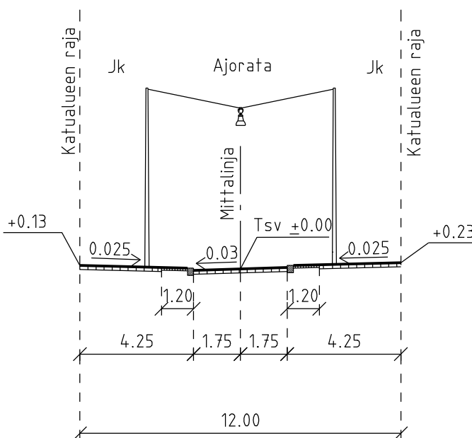
POIKKILEIKKAUS A-A 1:200
