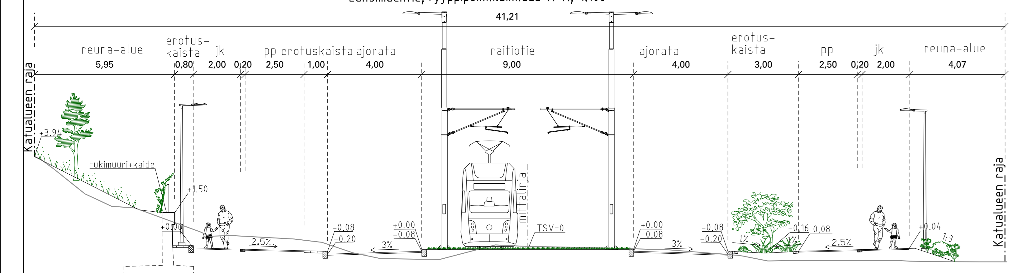
Länsimäentie, Tyypipoikkeilu C-C, 1:100
