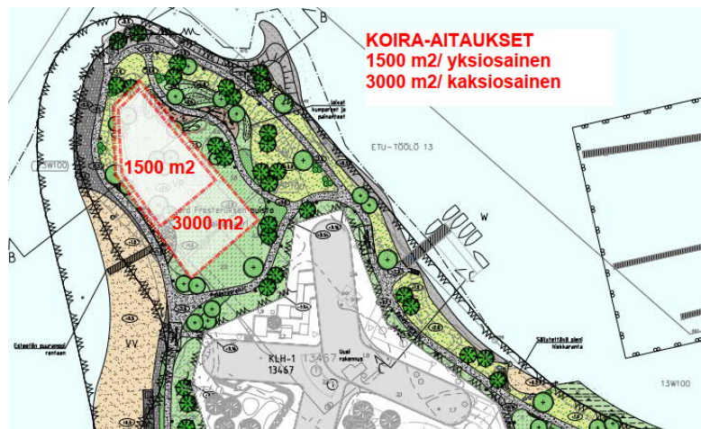
Kuva: Koira-aitauksen tilantarve. Yksiosainen esim. vain pienet koirat 1500, kaksiosainen jossa ovat osastot isoille ja pienille koirille yht. 3000mm.
