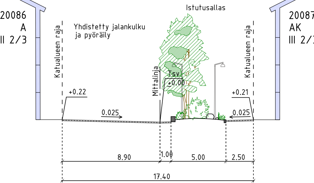
SAMOANKUJA LEIKKAUS A-A 1:200
