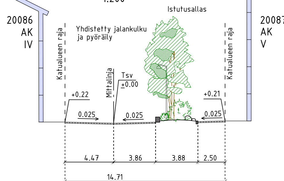
SAMOANKUJA LEIKKAUS B-B 1:200
