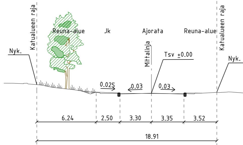
POIKKILEIKKAUS A-A, 1:200
