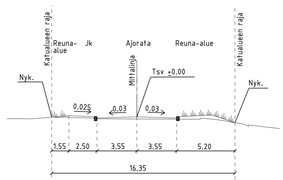
POIKKILEIKKAUS A-A, 1:200
