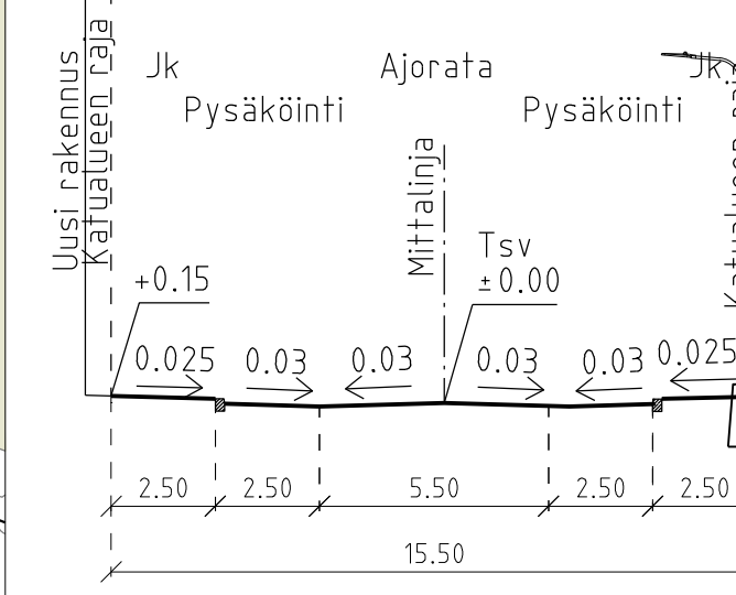
POIKKILEIKKAUS K-K 1:200
