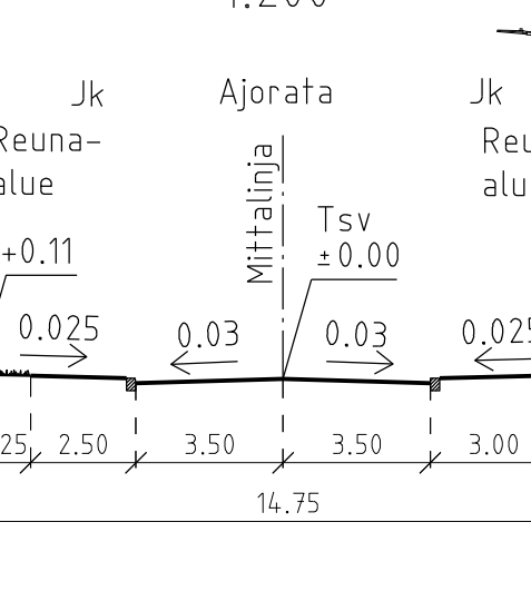
POIKKILEIKKAUS L-L 1:200
