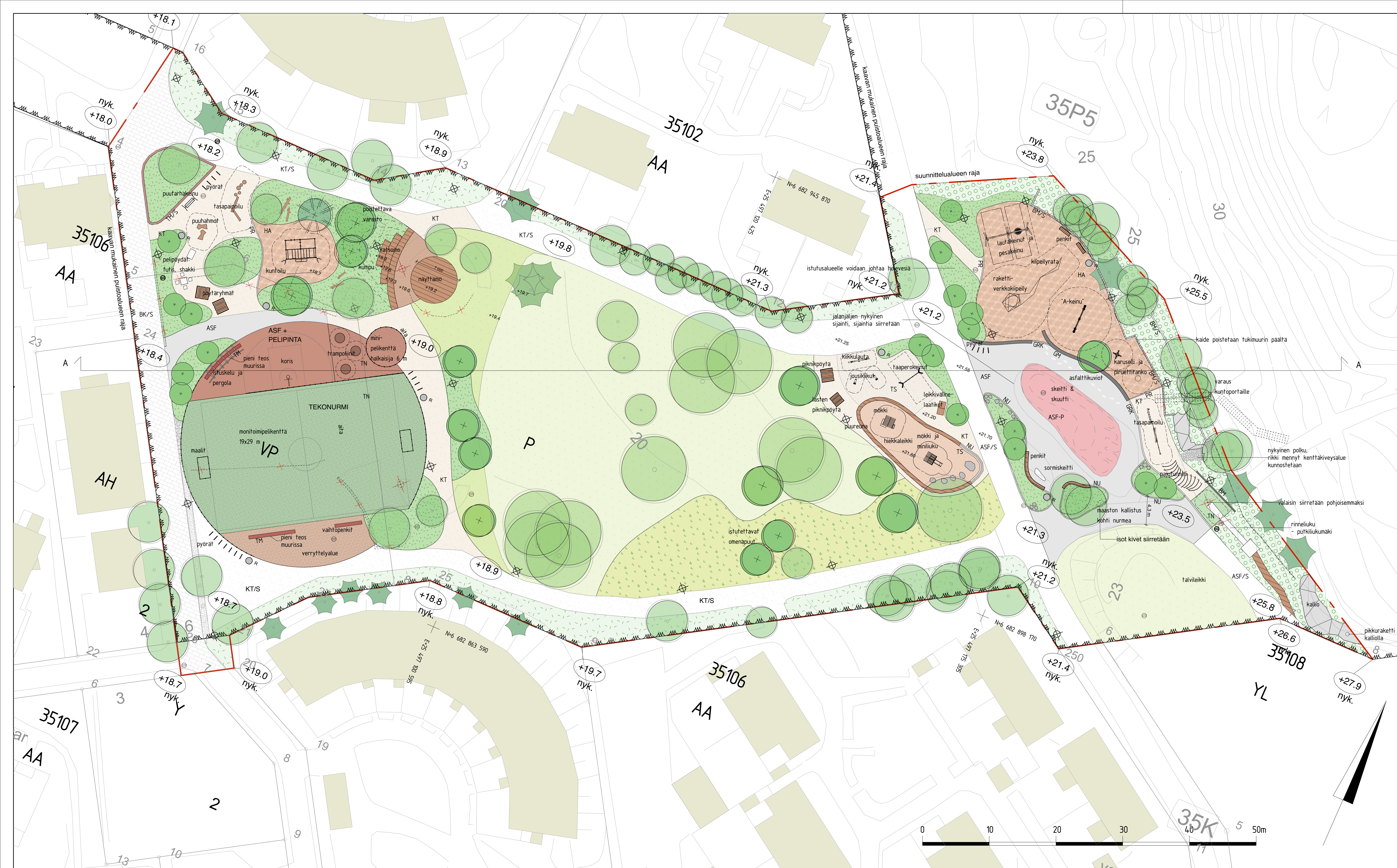
Puistosuunnitelma 1:200
