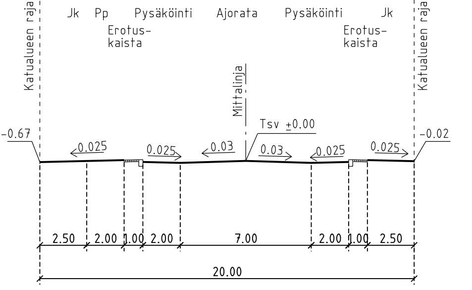
POIKKILEIKKAUS B-B 1:200
