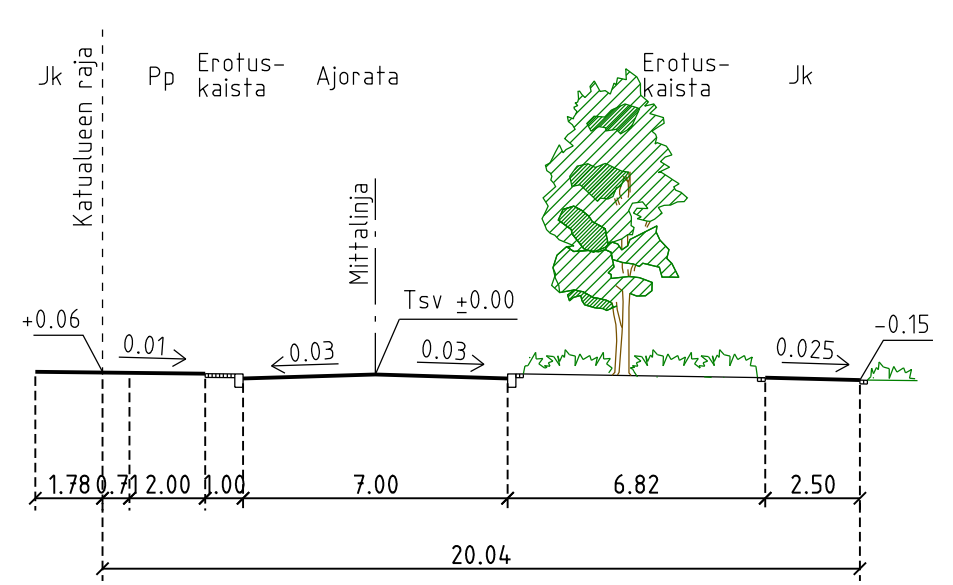
POIKKILEIKKAUS C-C 1:200
