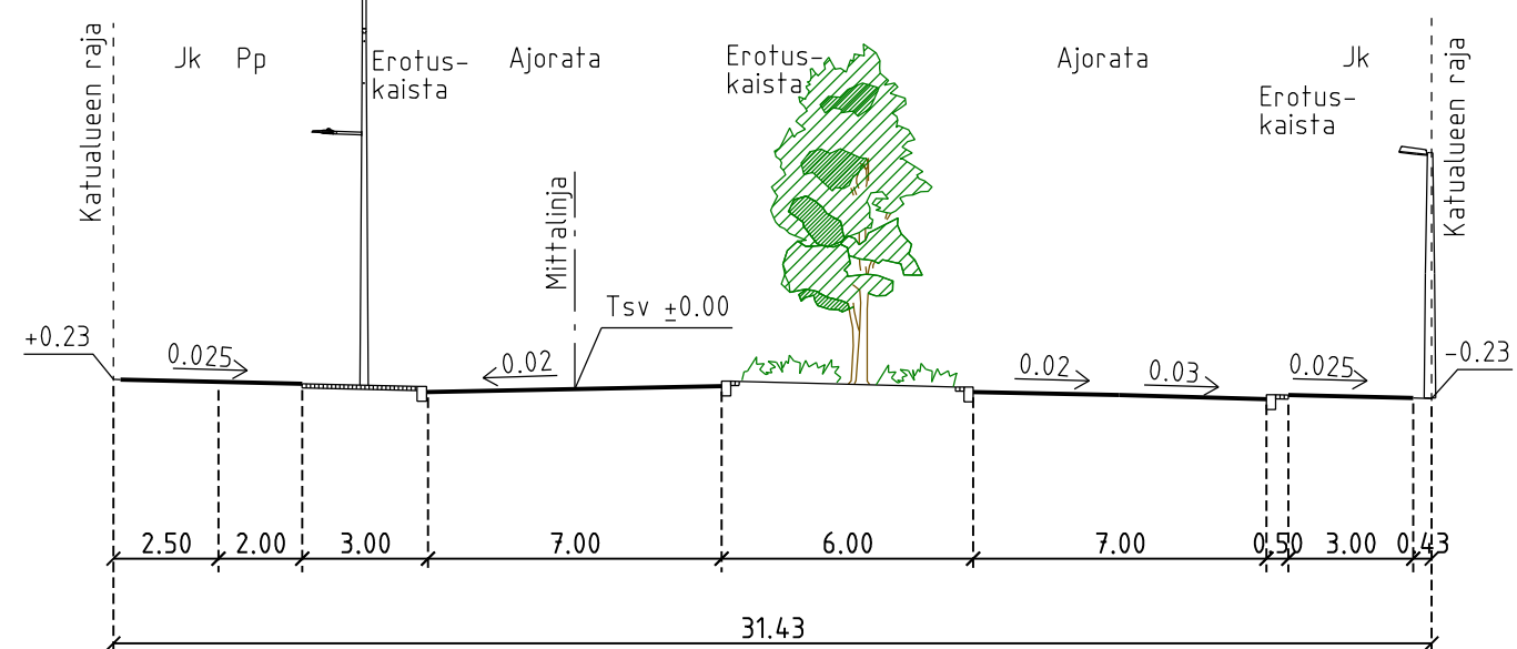
POIKKILEIKKAUS A-A 1:200
