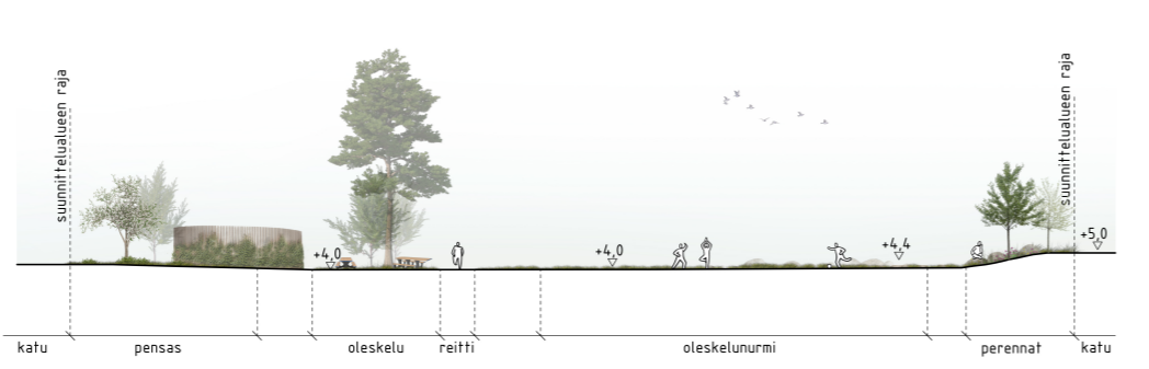
LEIKKAUS BB
