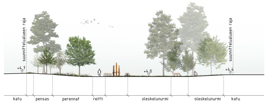
LEIKKAUS AA
