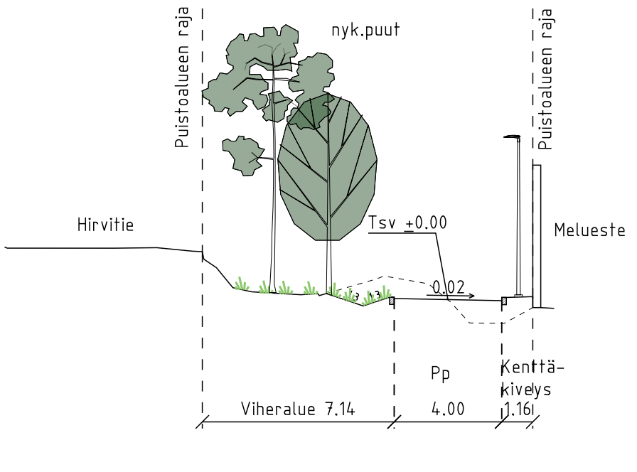
POIKKILEIKKAUS D-D PL. 530 1:200
