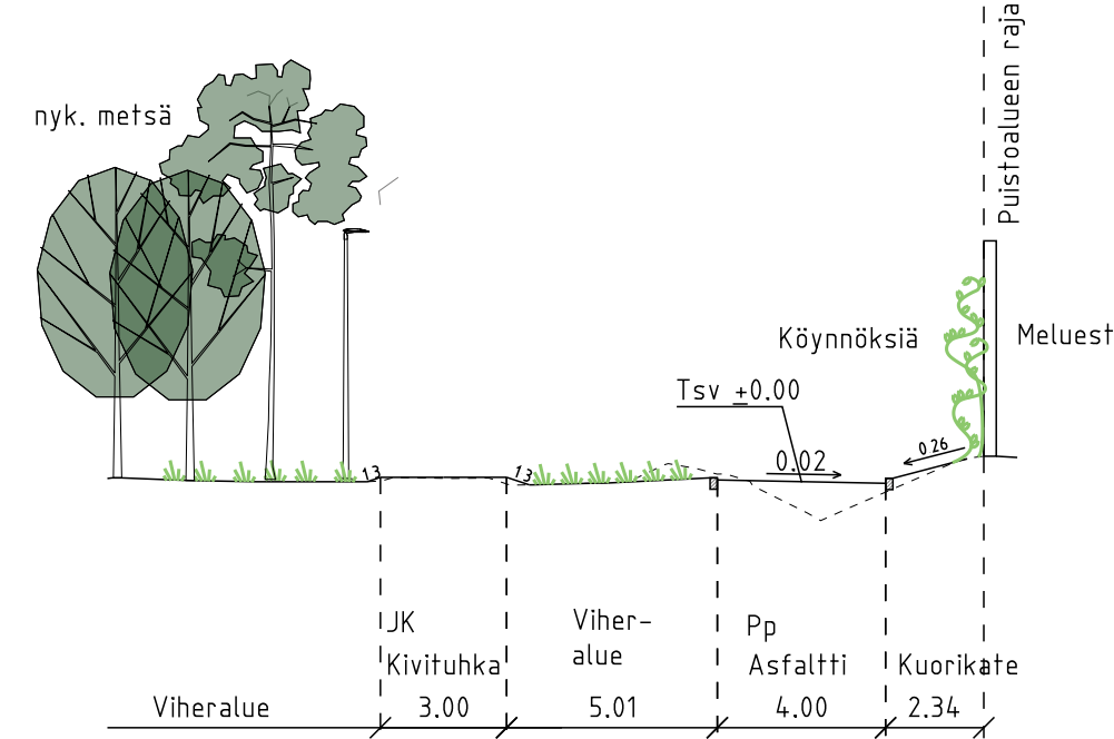
POIKKILEIKKAUS E-E PL. 735 1:200
