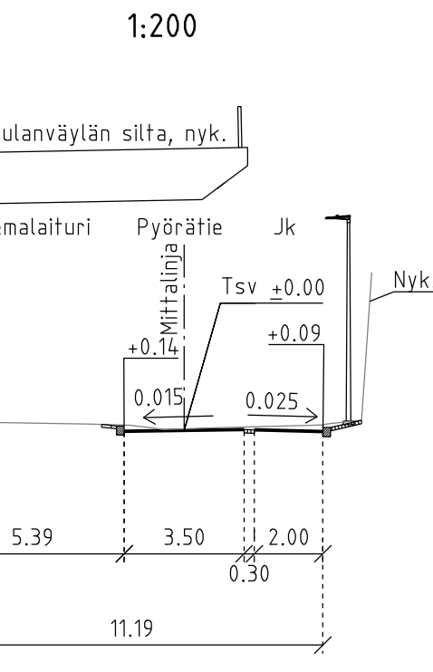
POIKKILEIKKAUS C-C 1:200
