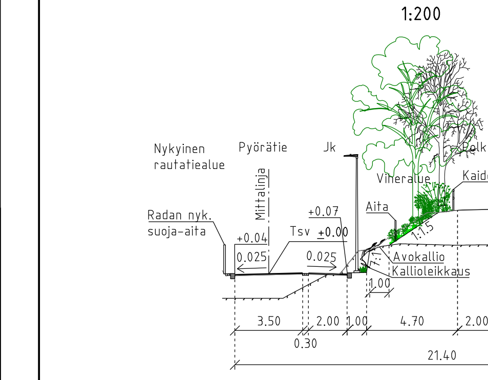
POIKKILEIKKAUS A-A 1:200
