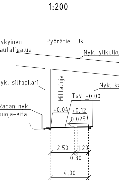
POIKKILEIKKAUS B-B 1:200
