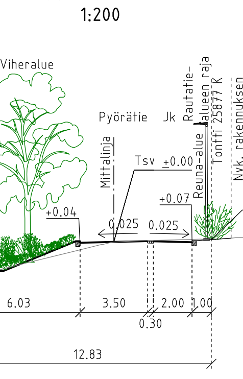
POIKKILEIKKAUS D-D 1:200
